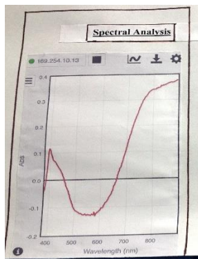
Cu(NO 3 ) 2 Spectrum
