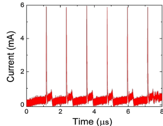
Spiking in a VO 2 nano “neuristor”
